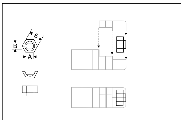
Elément d'insertion
